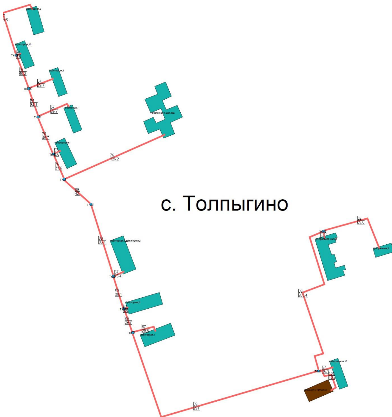
Рисунок 1.3.2.2 - Схема тепловой сети от Котельной с. Толпыгино
